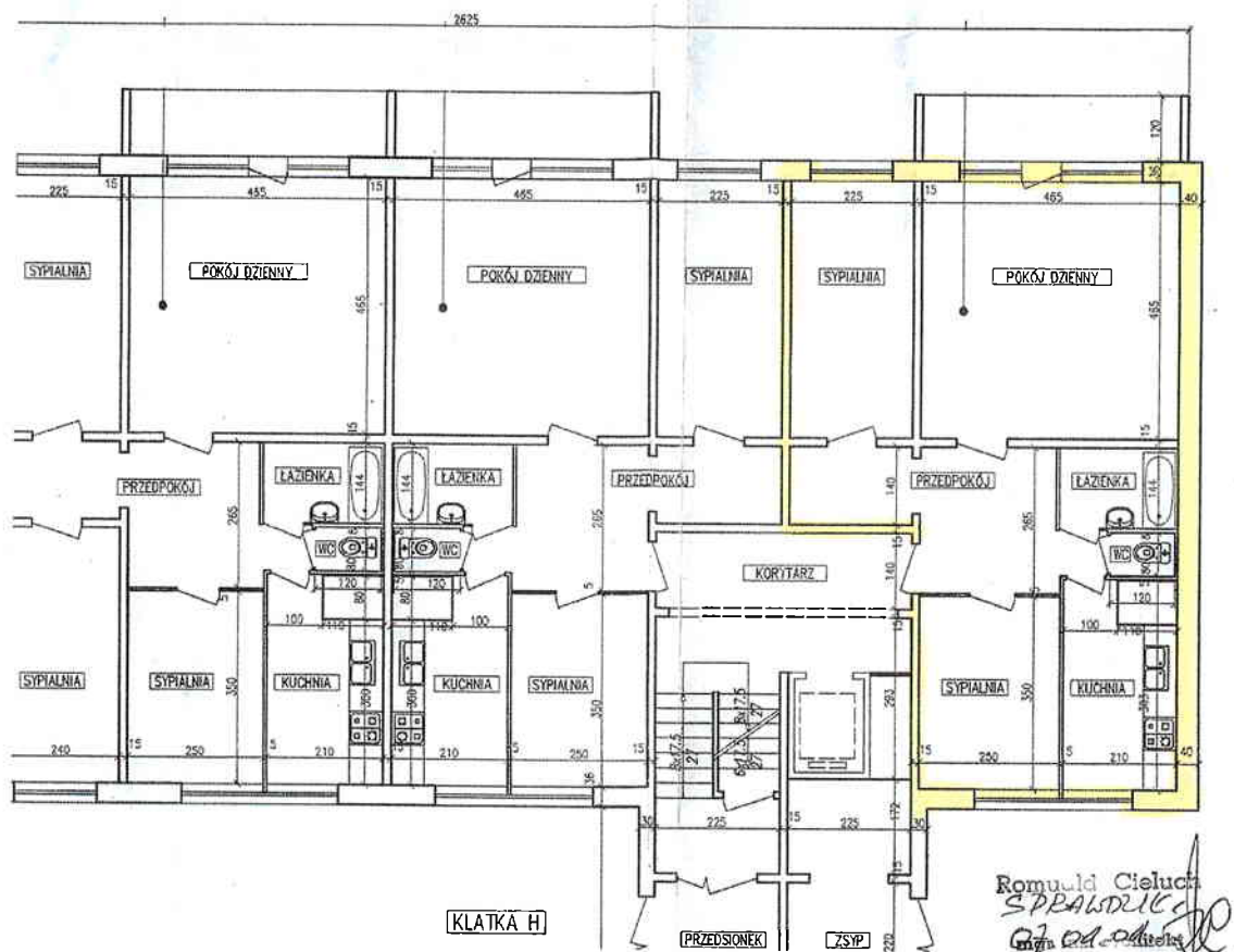
Mieszkanie skrajne w budynku (ze ścianą szczytową, zewnętrzną)
