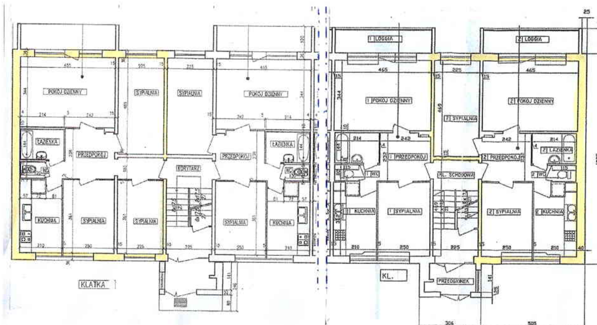
Mieszkania skrajne w budynku (ze ścianą szczytową ,zewnętrzną)
